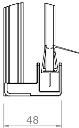
DETTAGLIO A SCALA 1 : 2
