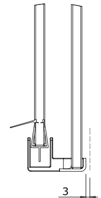
DETTAGLIO S SCALA 1 : 2
