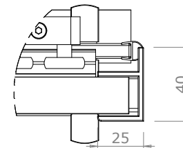
DETTAGLIO P SCALA 1 : 2
