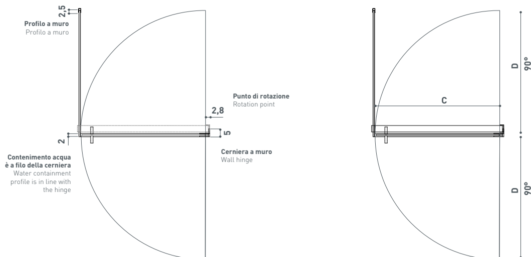
Sezione a 100 cm Section at 100 cm
