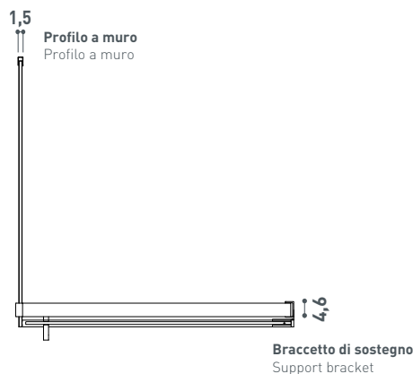
Sezione a 100 cm Section at 100 cm
