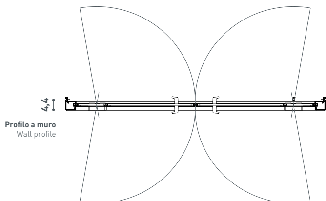
4,4 Profilo a muro Wall profile
