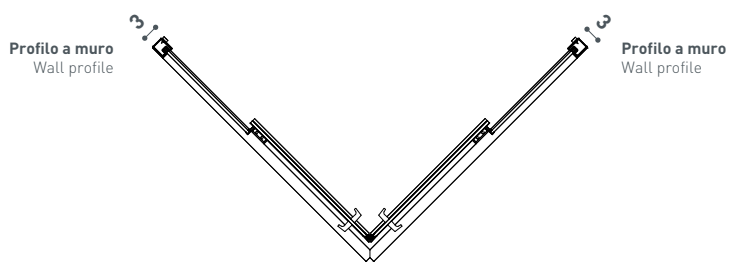
Sezione a 100 cm Section at 100 cm
